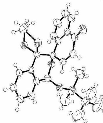
Figure 1. Crystal structure of 12a (ORTEP plot).
